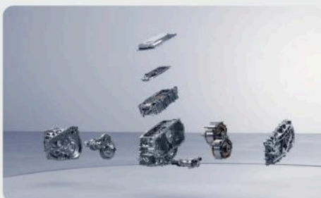
Hybrydowy napęd elektryczny 11in1 E-DHT
